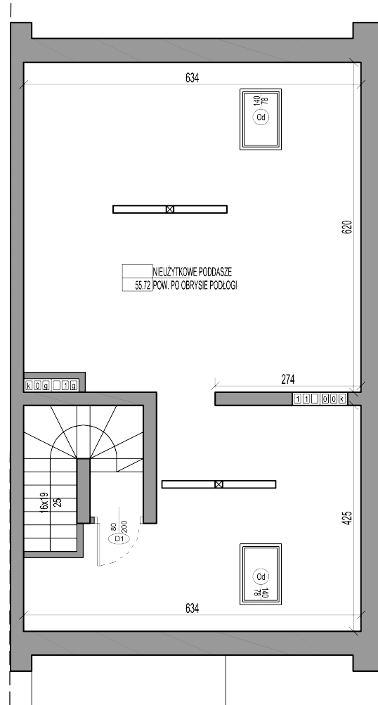
RZUT PODDASZA NIEUŻYTKOW. LOKAL 2
