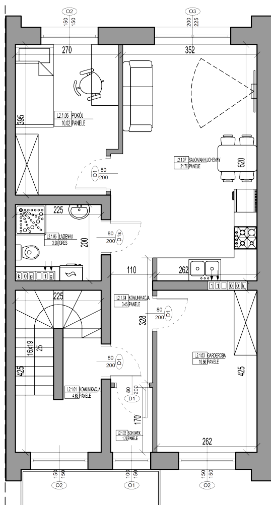
RZUT PIĘTRA LOKAL 2
